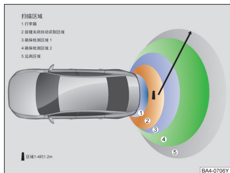
图 59 感应式行李厢盖开启和关闭钥匙有效识别区域
