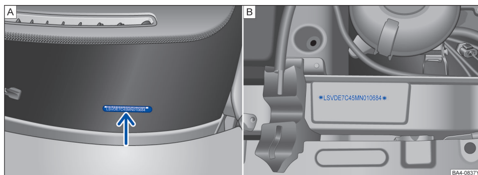
图 212 [A]. 车辆识别代号。[B]. 发动机舱内的车辆识别号钢印位置
