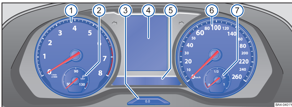
图 9 多功能组合仪表
