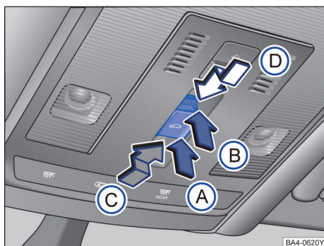
图 65 顶篷上的天窗控制按钮
