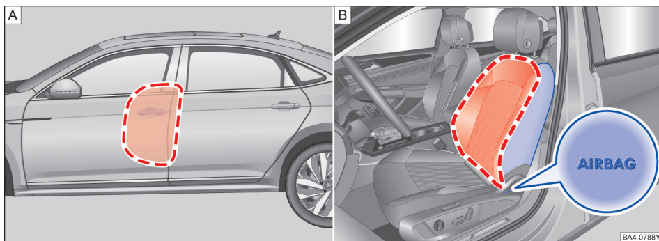
图 37 [A] 轿车左侧 - 侧面安全气囊膨胀范围；[B] 左前座椅侧面 - 侧面安全气囊安装位置及膨胀范围
