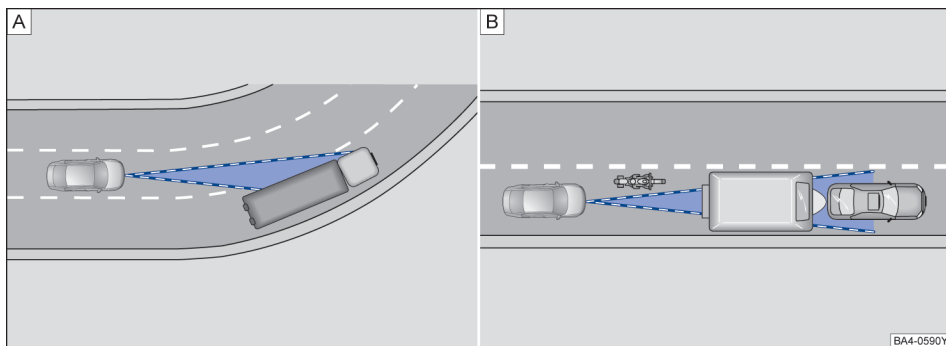
图 124 A 处在弯道里的轿车；B 前方行驶的摩托车处在雷达传感器探测范围外
