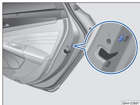
图 53 右侧后车门端面处的应急上锁装置（由橡胶密封件遮盖着）
