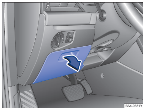
图 181 在驾驶员侧仪表板上：保险丝盒盖板
