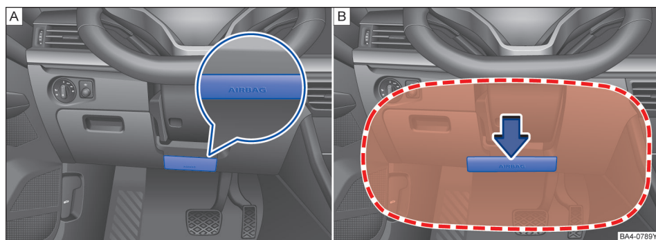
图 39 驾驶员侧：膝部安全气囊安装位置及作用范围
