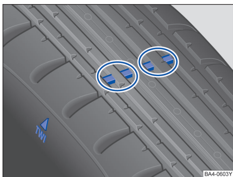
图 199 轮胎花纹磨损标记
