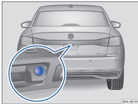
图 144 车辆行李厢盖内：倒车摄像头的安装位置
