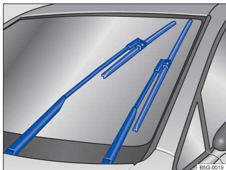
图 93 车窗玻璃刮水器在维护位置
