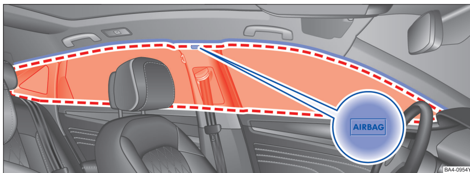
图 38 在汽车左侧：头部安全气囊的安装位置和膨胀范围
