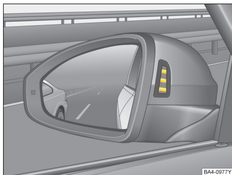
图 132 车外后视镜外壳内：变道辅助系统的可视显示
