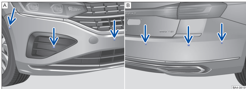
图 137 前后保险杠：泊车雷达系统超声波传感器
