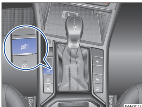
图 134 在中控台：自动驻车功能按钮
