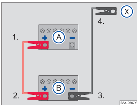
图 183 跨接电缆连接示意图
