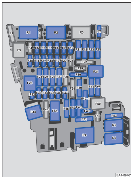
图 182 保险丝位置示意图
