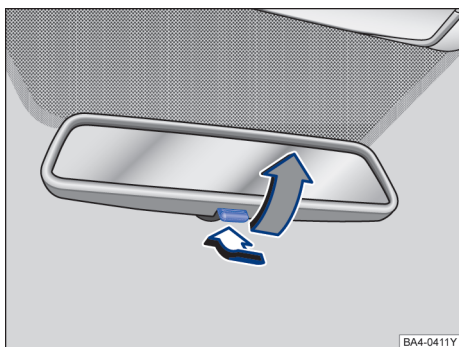
图 96 手动防眩车内后视镜
