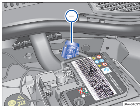
图 184 用于充电器负极连接的接地点
