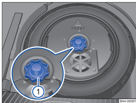
图 202 行李厢内：备用车轮（类型 B）固定手轮
