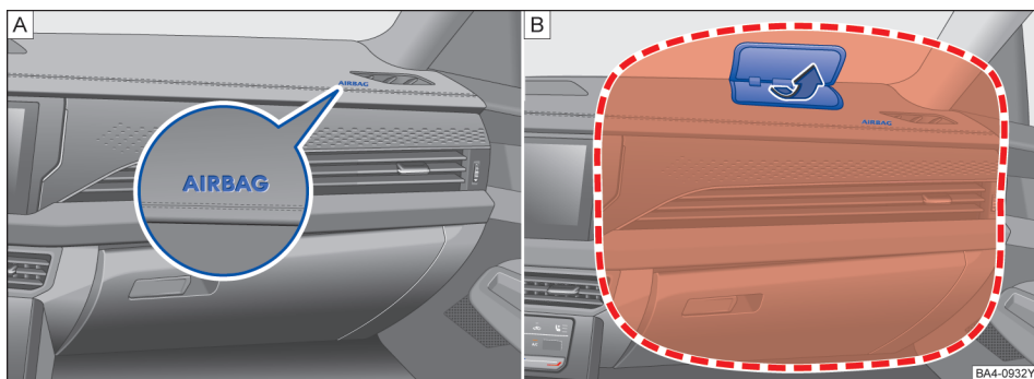
图 36 副驾驶员前部安全气囊的安装位置和膨胀范围
